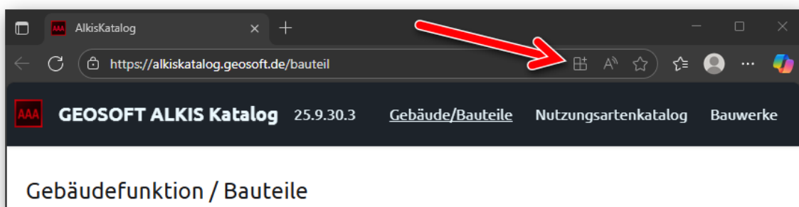
Abbildung 2: Installationsmenü aufrufen
